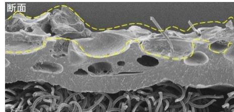
旧スベリ止め（マイクロフィニッシュ）断面図
