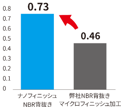
摩擦係数試験結果（グリップ力の測定）
