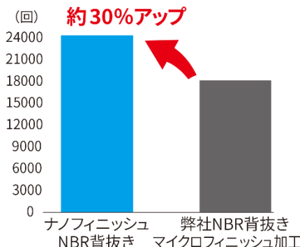
磨耗強度試験結果
